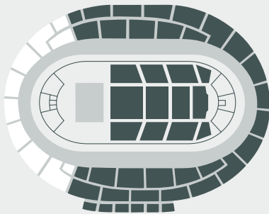
1. Reihenbestuhlung mit Front-Bühne Bühnenfläche: 26 m x 16 m Kapazität: ca. 7.000
